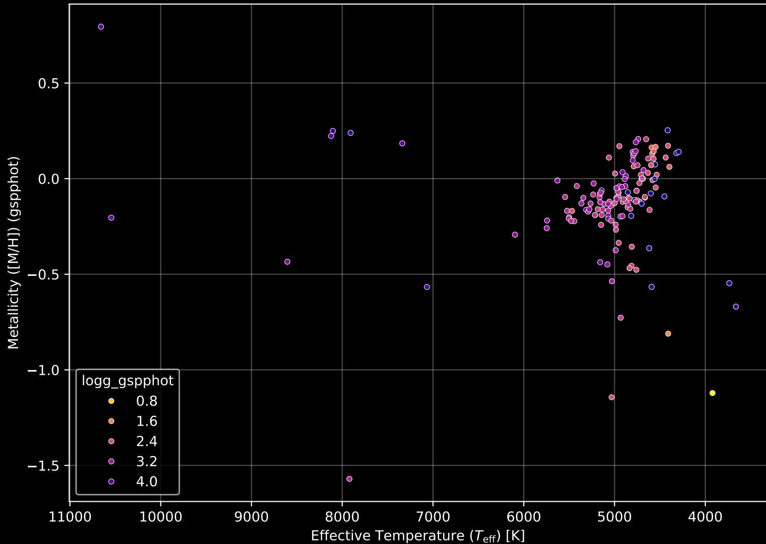
APOGEE DR17 Field: [188-12] Stellar Population Parameters (n= 142)
